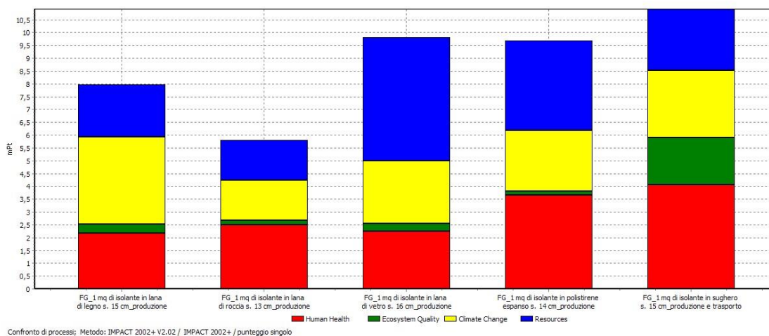
Comparazione LCA tra diversi strati di isolamento termico
